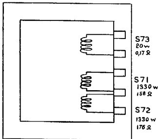
VOEDING TRAF0 GK 512 71
