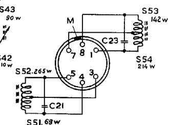
M.F. SPOEL II GK 563 83
