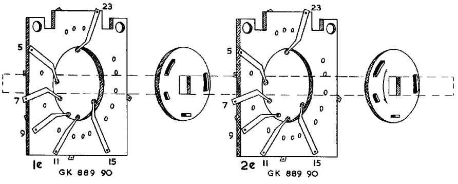
DE TWEE SEGMENTEN DER GOLFBEREIKSCHAKELAAR, NAAR DE KNOP TOEGEZIEN
