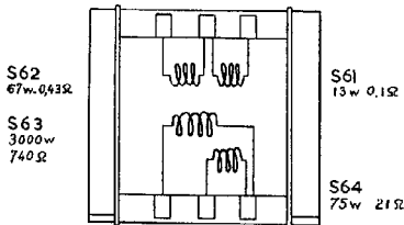
UITGANG TRAF0 GK 512 73
