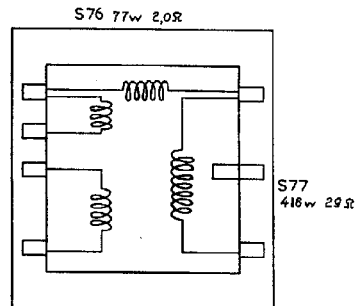
VOEDING TRAF0 GK 512 71
