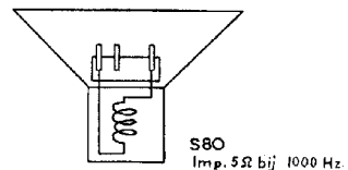
SPREEK SPOEL LUIDSPREKER 49 238 36
