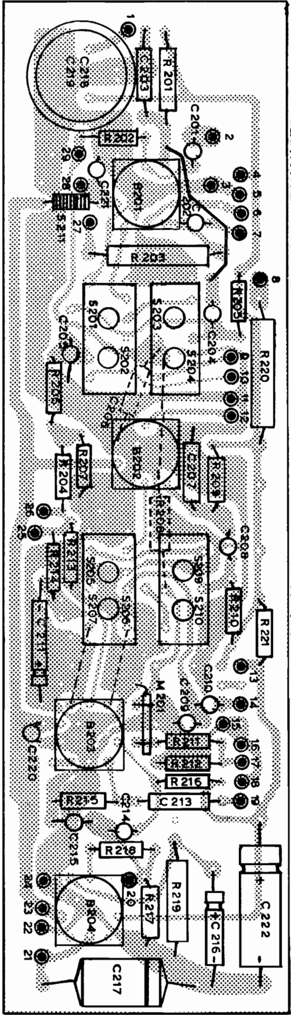
GEDRUKTE BEDRADING
